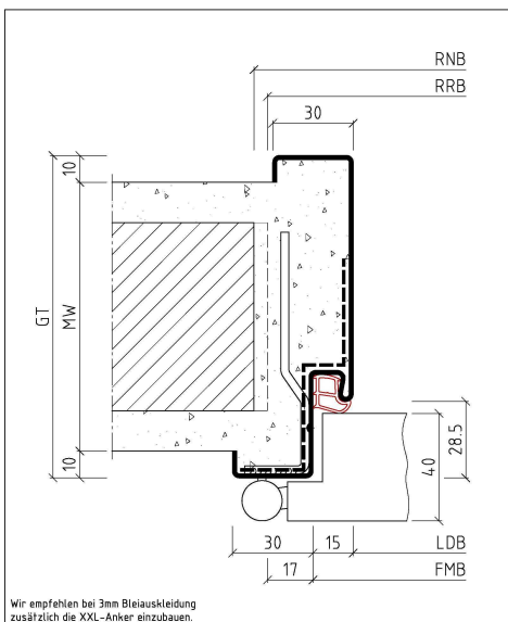
Mauerwerkszarge
