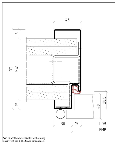
Ständerwerkszarge
