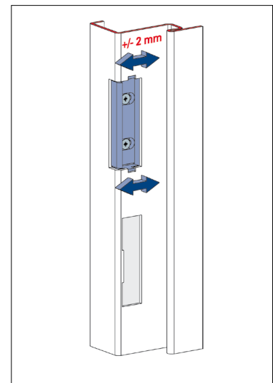
Mit wenigen Handgriffen vor Ort einstellbar: BOS-Fallenverstellung.
